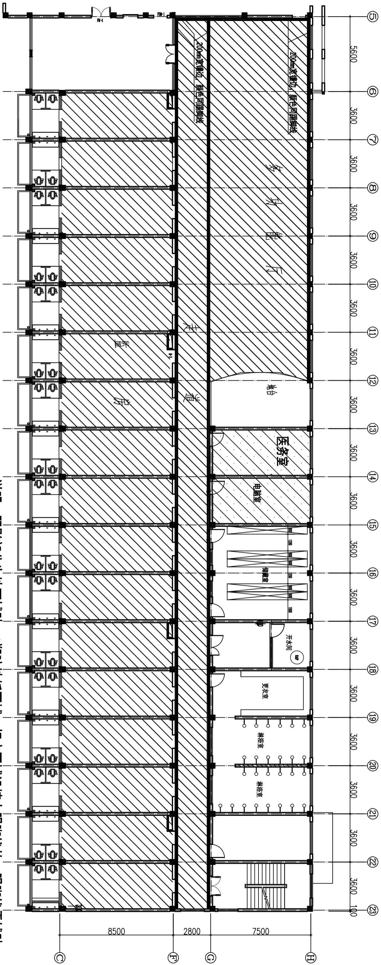
施工区域平面图
